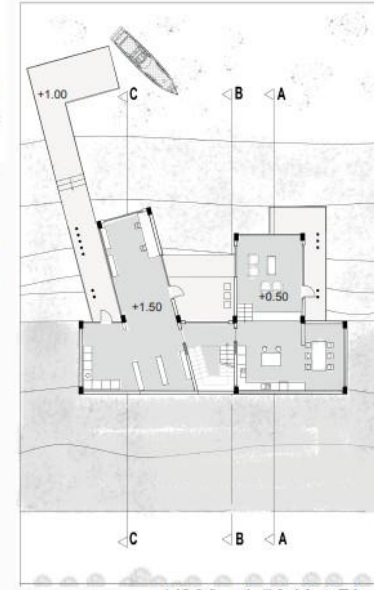
1/200 +1.50 Kot Planı
